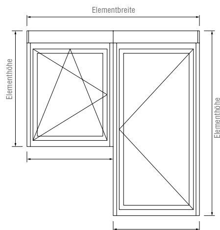
Kombi-Element Fenster/Tür
