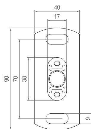
Klemmkonsole KK40
