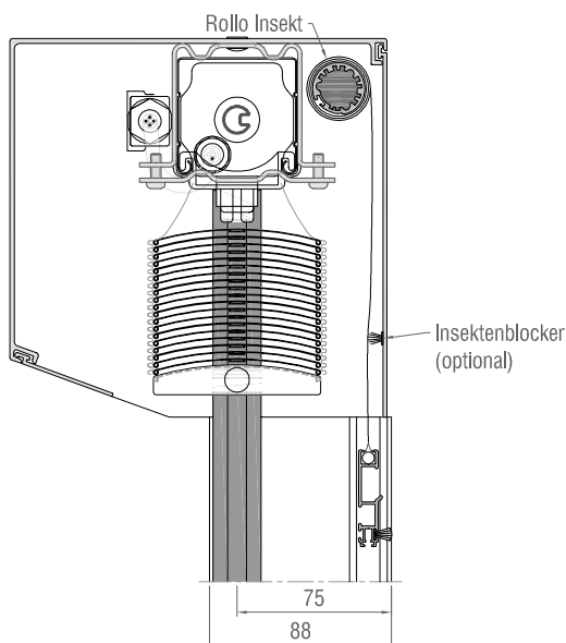
Vorbaukasten
