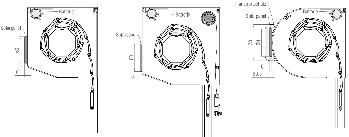
Detail Solarpanel auf gerader Blende montiert.
