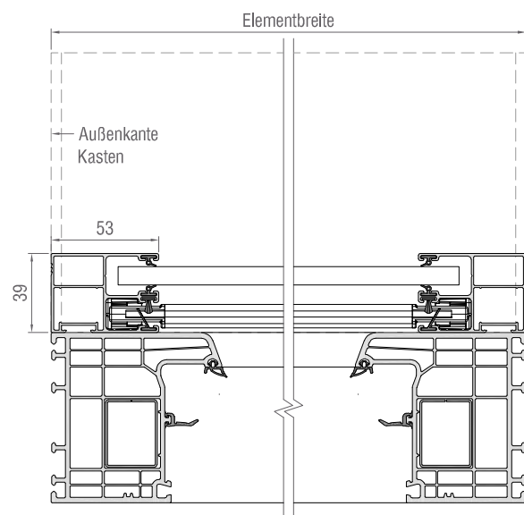
Führungsschienen-Querschnitt
