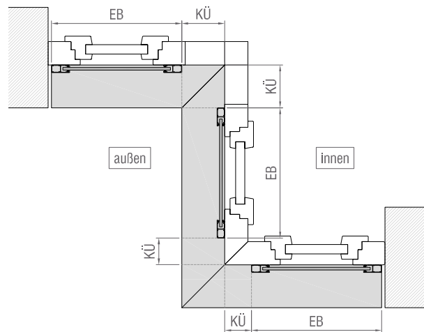
Innen-Außen-Kombination
