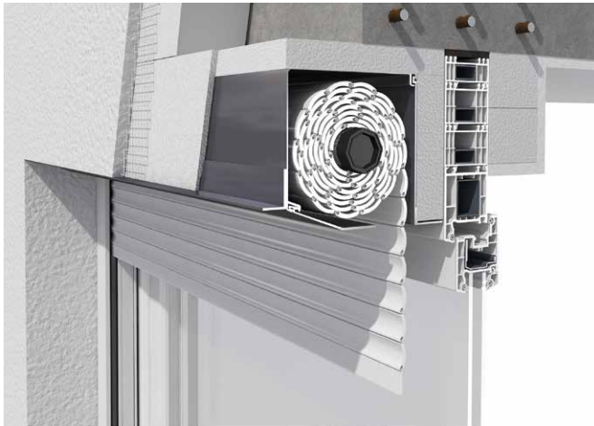
Einbausituation Putzträgerkasten stranggepresst 20°
