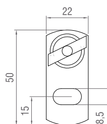
Abstandshalter HE70
