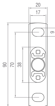
Klemmkonsole KK20
