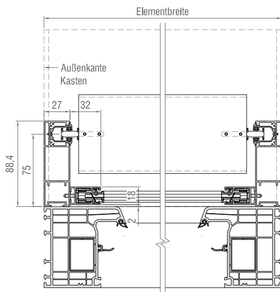
Führungsschiene-Querschnitt
