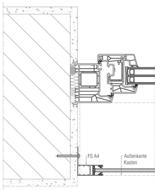
Detail Führungsschiene
