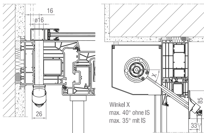
Kurbelabgang schräg 40°
