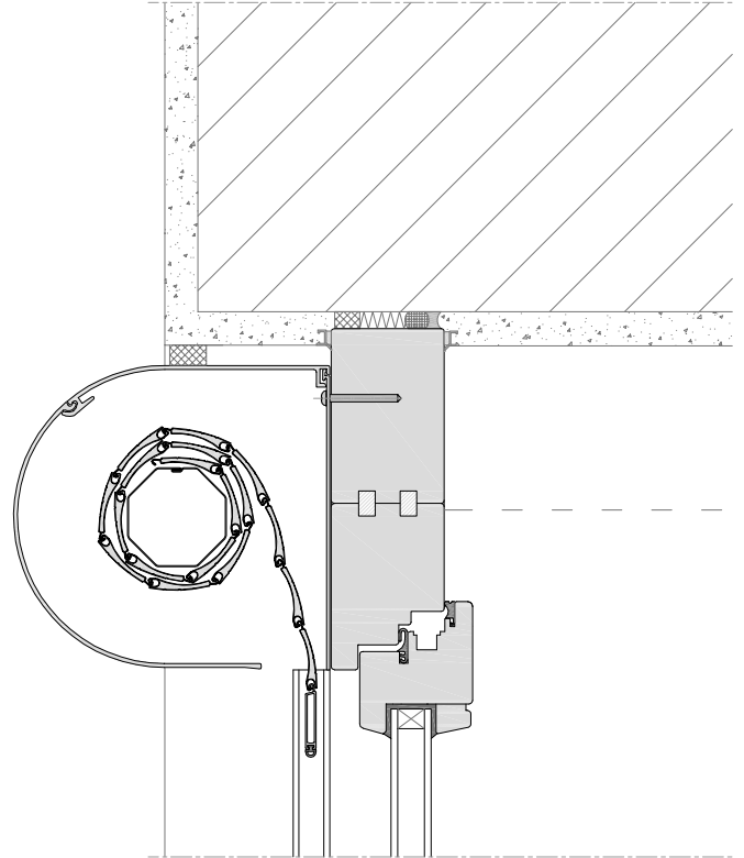
Kastenbefestigung innen
