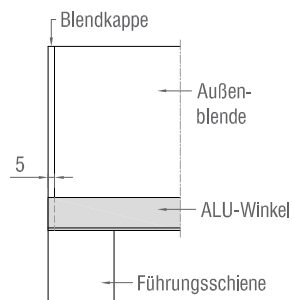
Detail Kastenabschlussprofil, Ansicht von vorn Putzträgerkasten eckig 90° mit ALU-Winkel
