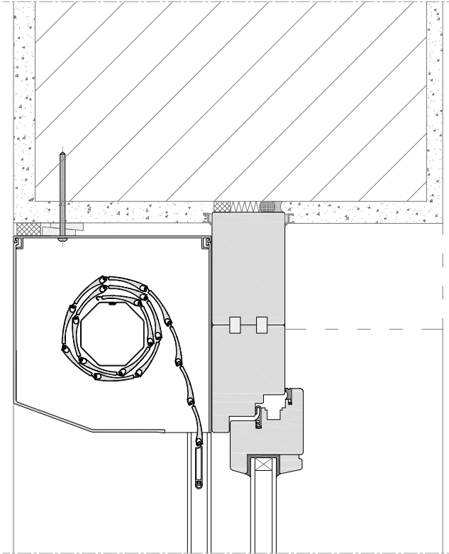
Kastenbefestigung oben
