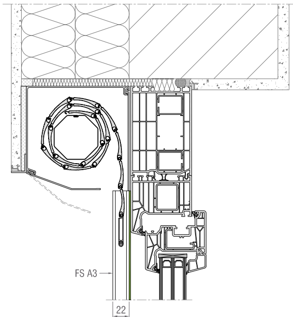
Darstellung am Beispiel A3 Führungsschiene mit schlagregendichter Abdichtung
